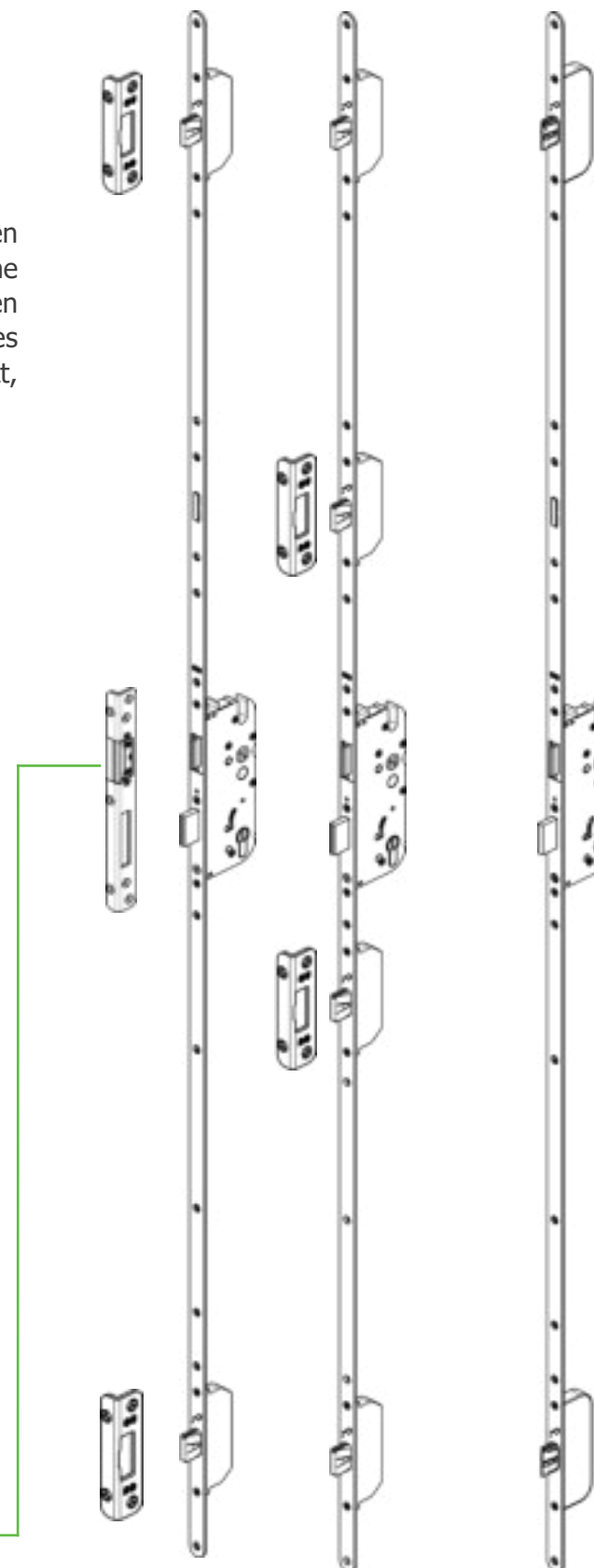
Manuelle Dreifach- oder Fünffachverriegelung optional mit E-Öffner
